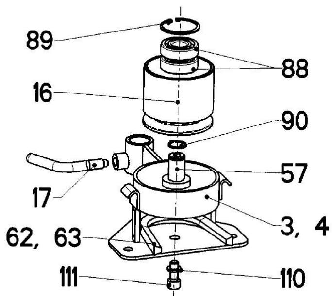
Spojka typ VARI, Honda – průměr 80mm
